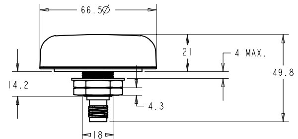
TW3870/TW3872 Dimensions (mm)
